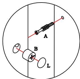
Detalhe da fixação do Minifix.
