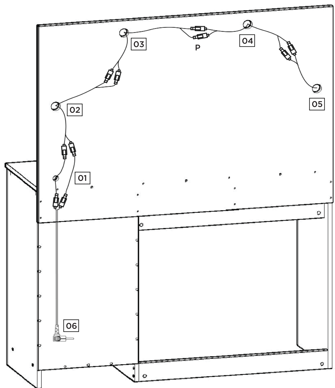
Detalhe da fiação do Kit Luminária Led.
