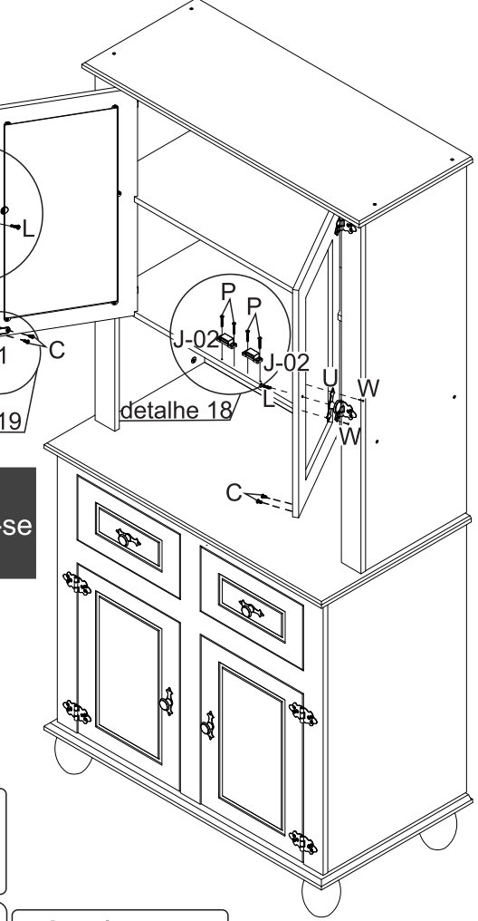
L- Parafuso MQ FL M4x22 OV (2x)
