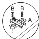
Detalhe fixação do calço na lateral
