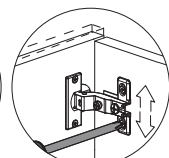
Regulagem para cima/para baixo
