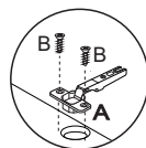
Detalhe fixação da dobradiça na porta
