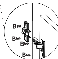
Detalhe da fixação da dobradiça (A) nas portas e laterais
