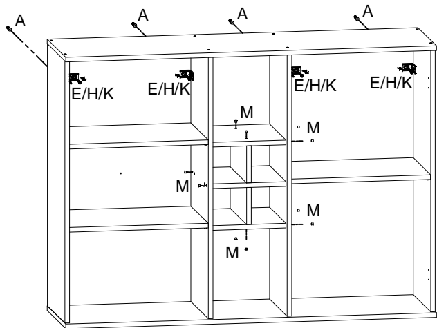
4º passo - Fixar suportes aéro, buchas na parede e colocar tapas furos
