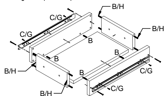
Montagem do porta tempero
