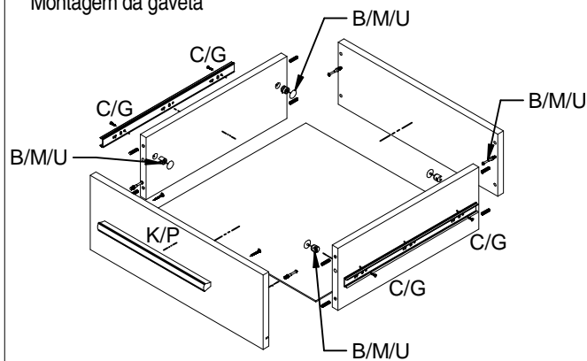
Montagem da gaveta
