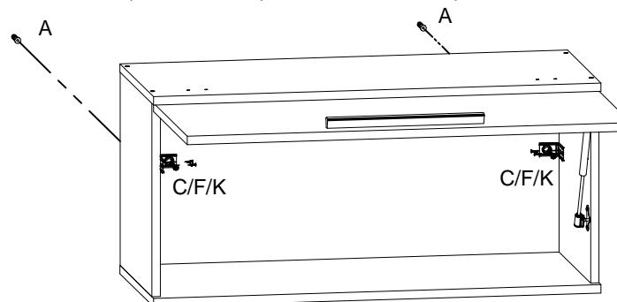
6º passo - Fixar suporte aéreo e buchas na parede
