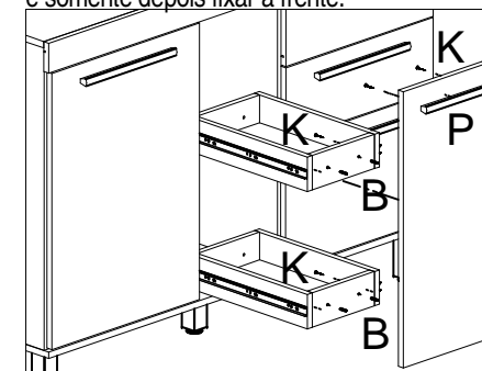
Fixação da frente do porta tempero Obs. colocar primeiro o porta tempero e somente depois fixar a frente.
