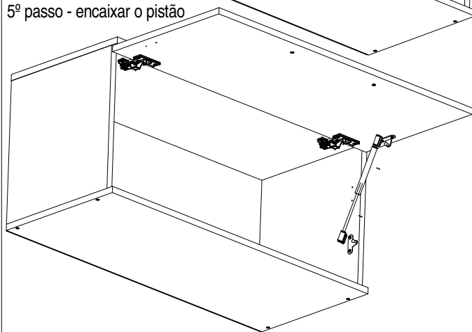
5º passo - encaixar o pistão
