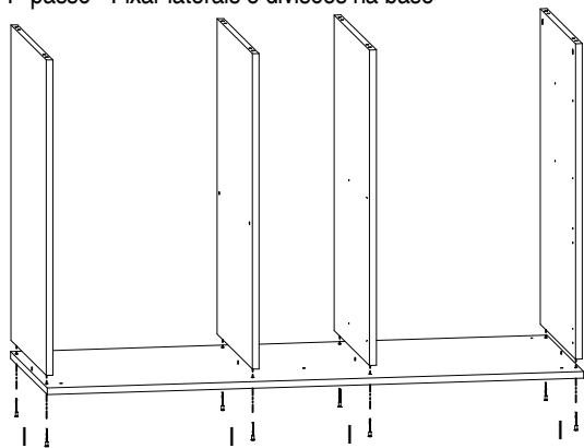
1º passo - Fixar laterais e divisões na base
