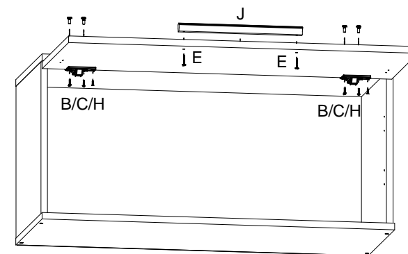
3º passo - Fixar porta e puxador
