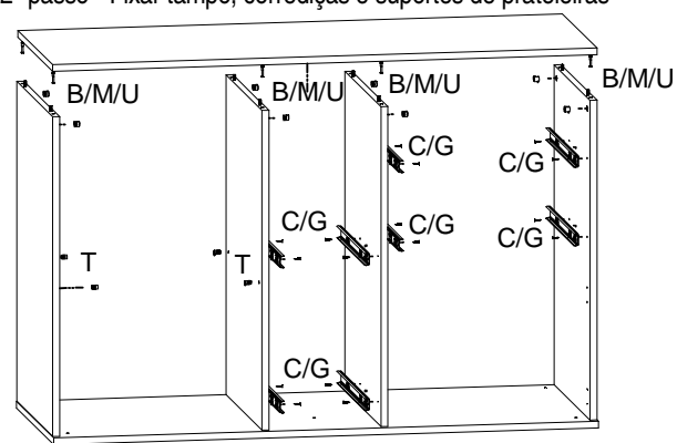
2º passo - Fixar tampo, corredeiras e suportes de prateleiras
