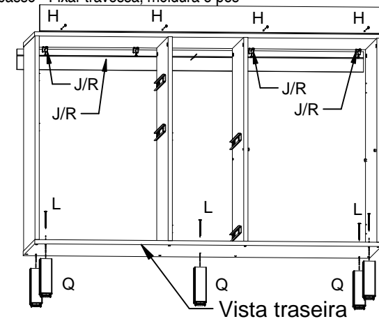
3º passo - Fixar travessa, moldura e pés
