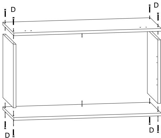
1º passo - Fixar base e tampo nas laterais
