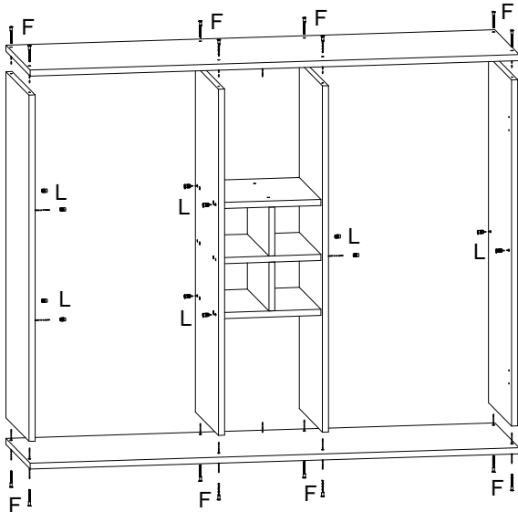
2º passo - Fixar as divisões e laterais na base e tampo
