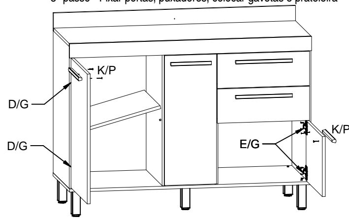
5º passo - Fixar portas, puxadores, colocar gavetas e prateleira
