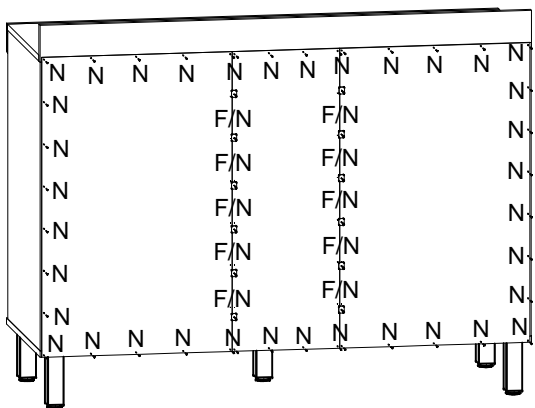
4º passo - Fixar fundos
