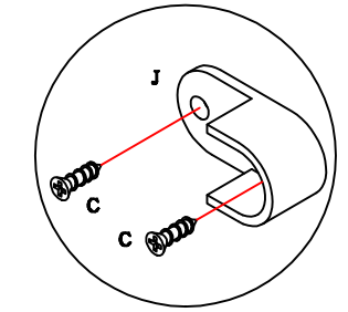
Detalhe da fixação do Minifix.
