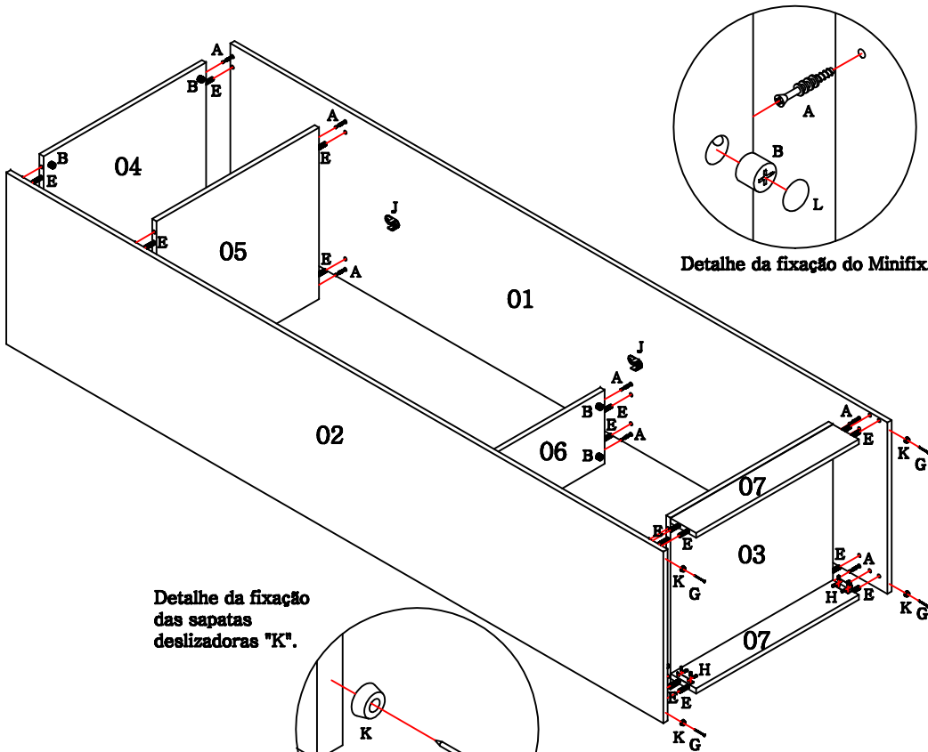
Fixe os rodapés com as cantoneiras "H" pelo lado interno.
