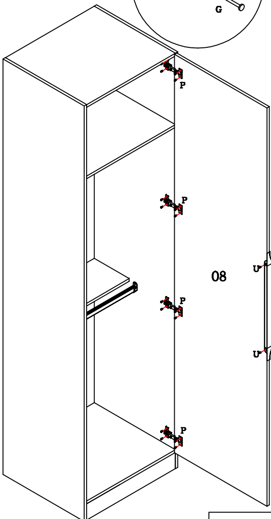
Utilize os parafusos "U" para fixar o puxador.
