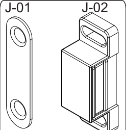
J- Fecho Magnético (SOPRANO) (2x)
