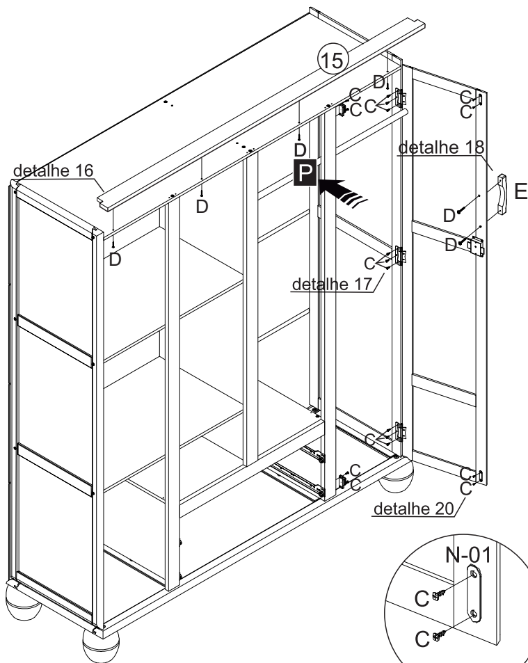
detalhe 20
