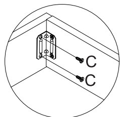
detalhe 22
