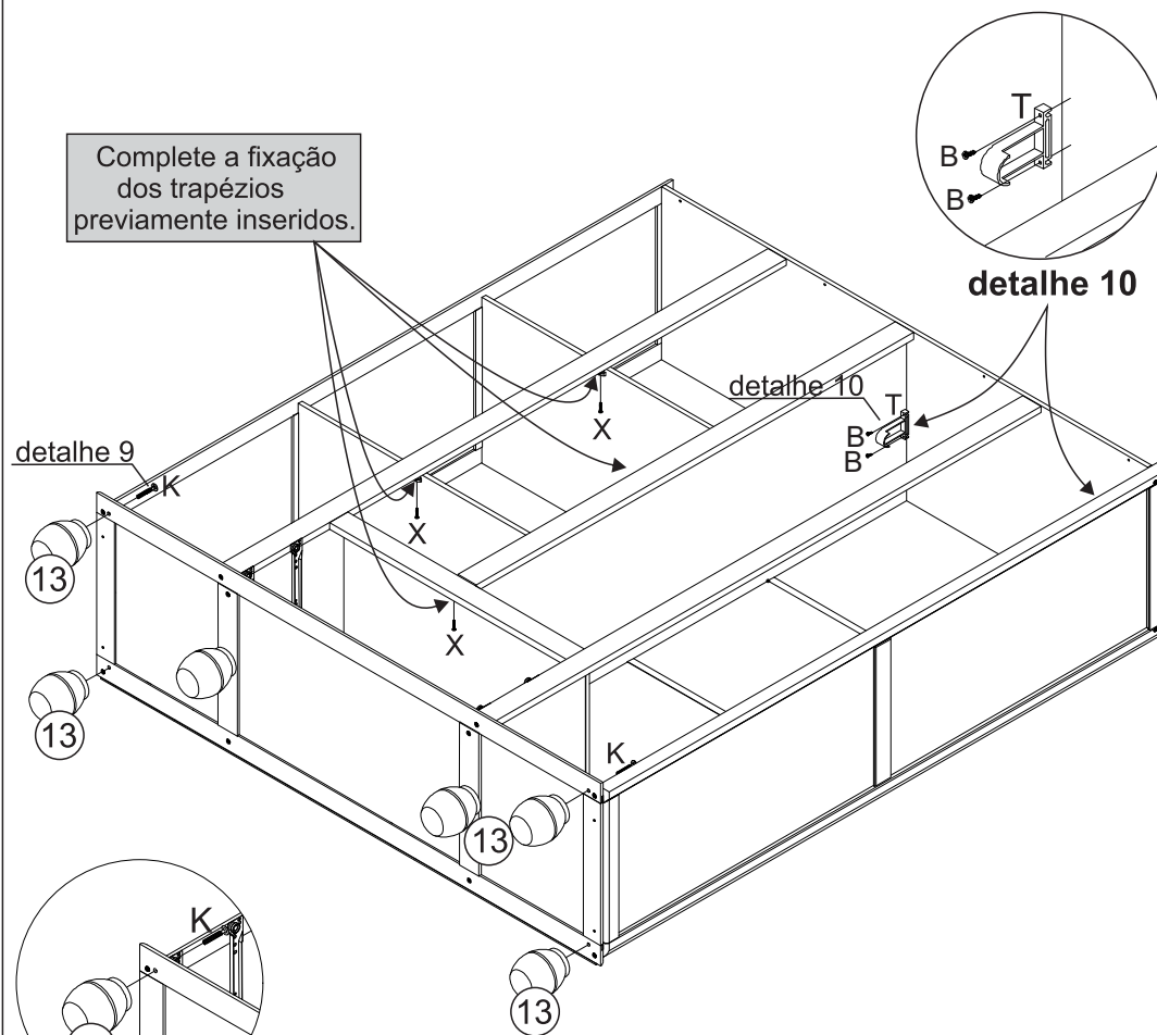
detalhe 9
