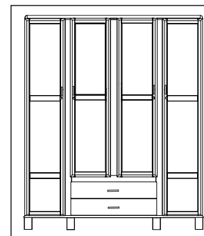
detalhe 17
