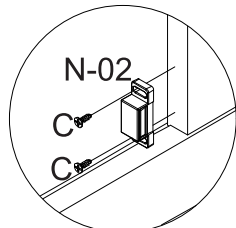
detalhe 19
