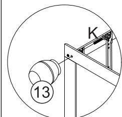
detalhe 9
