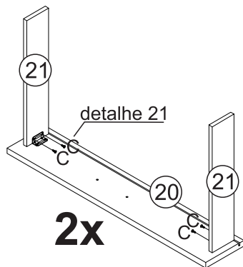
detalhe 21
