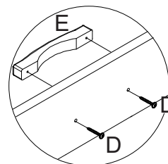
detalhe 24
