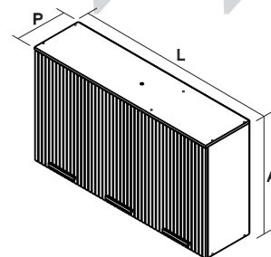
ARM 3PT-120 PRODUTO MONTADO: A: 690 L: 1200 P: 310 MM
