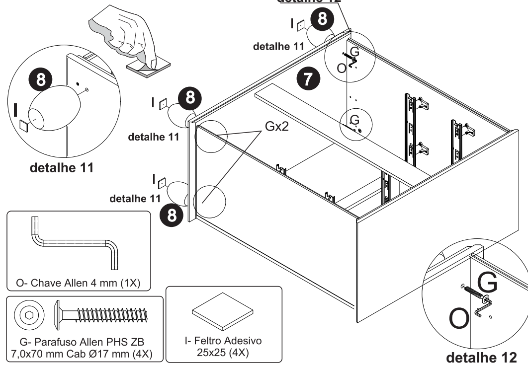
detalhe 12
