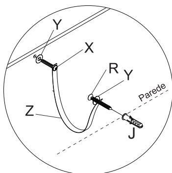
detalhe 18
