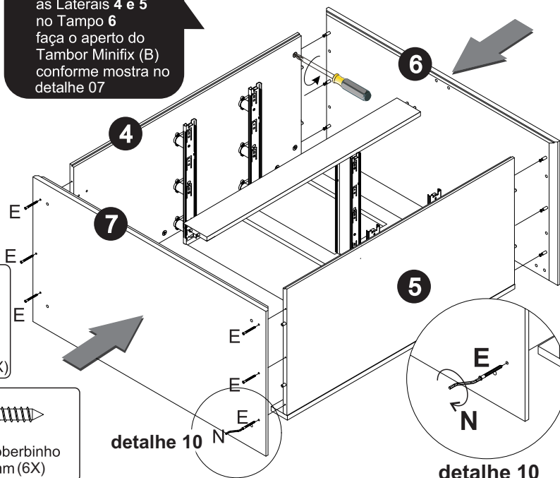
detalhe 10
