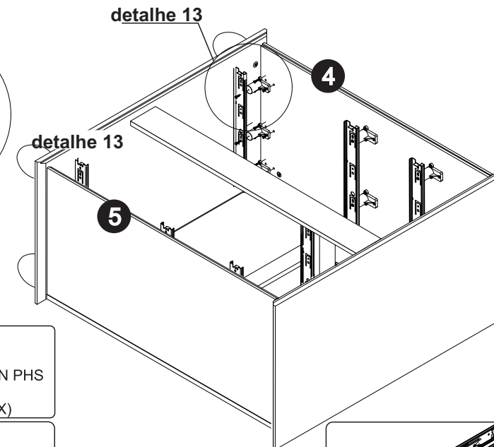
detalhe 13
