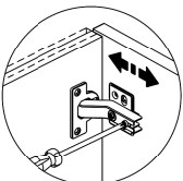
Regulagem Profundidade
