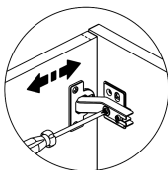
Regulagem Horizontal
