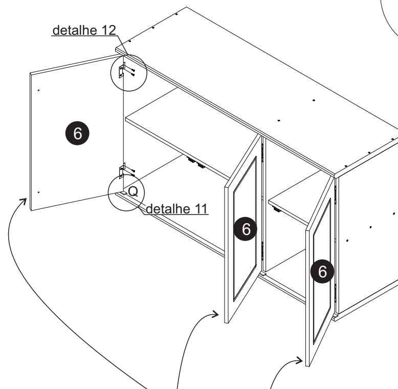
detalhe 12
