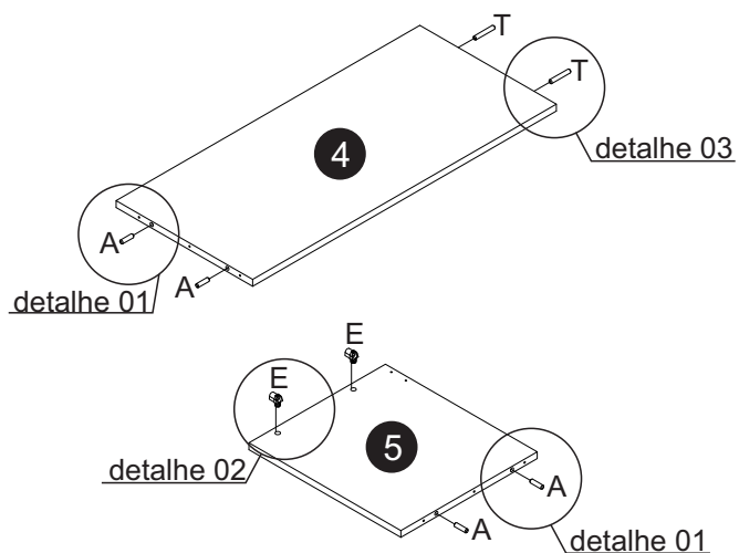
detalhe 01
