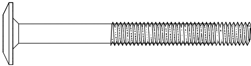
A- Parafuso Estrutural Allen ZB Ø1/4x60 mm CAB 13 mm (8x) COD 10476
