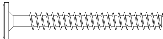
K- Parafuso estrutural ZP 7,0X50 sx interno cab. 17mm (4x) Cod 15892
