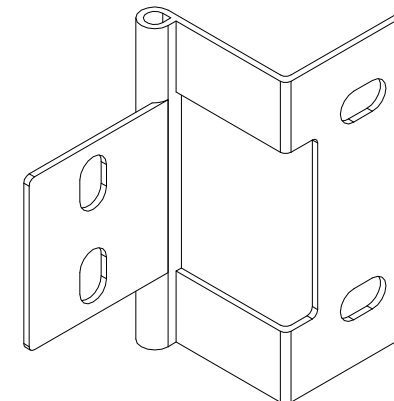
R- Dobradiça OV - JOY Cozinha (4x) Cod 48861
