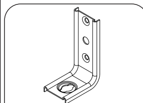
P- Cantoneira Metálica para fixação (3x)
