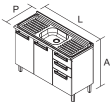
IG3G2-120 PIA PRODUTO MONTADO: A: 900 L: 1200 P: 500 MM
