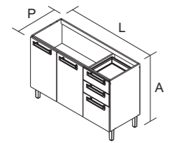
IG3G2ST-120 PRODUTO MONTADO: A: 830 L: 1200 P: 500 MM
