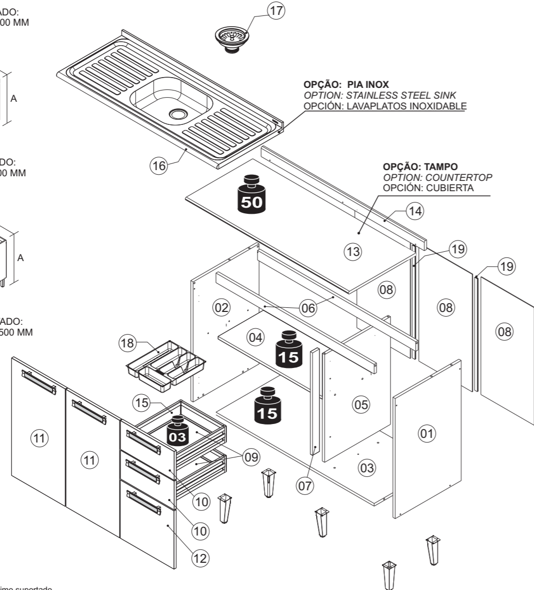
PUXADOR / DIMENSÃO HANDLE / DIMENSION TIRADOR / DIMENSIÓN
