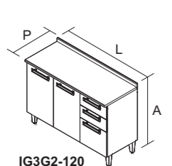
IG3G2-120 PRODUTO MONTADO: A: 900 L: 1200 P: 500 MM
