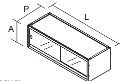
IPGV-70 PRODUTO MONTADO: A: 0,22 L: 0,70 P: 0,28 M
