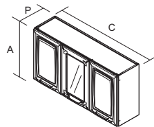
IP31V-105 MX Produto Montado C: 1050 mm A: 550 mm P: 280mm
