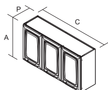
IP3-105 MX Produto Montado C: 1050 mm A: 550 mm P: 280mm
