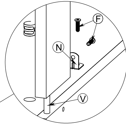
DETALHE B DETALLE B
